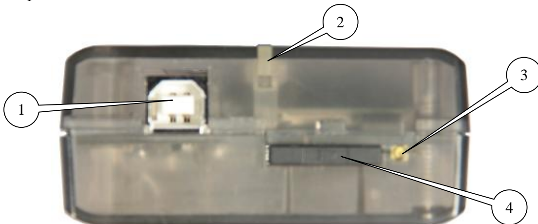
Рис.2.4.1 Вид спереди
